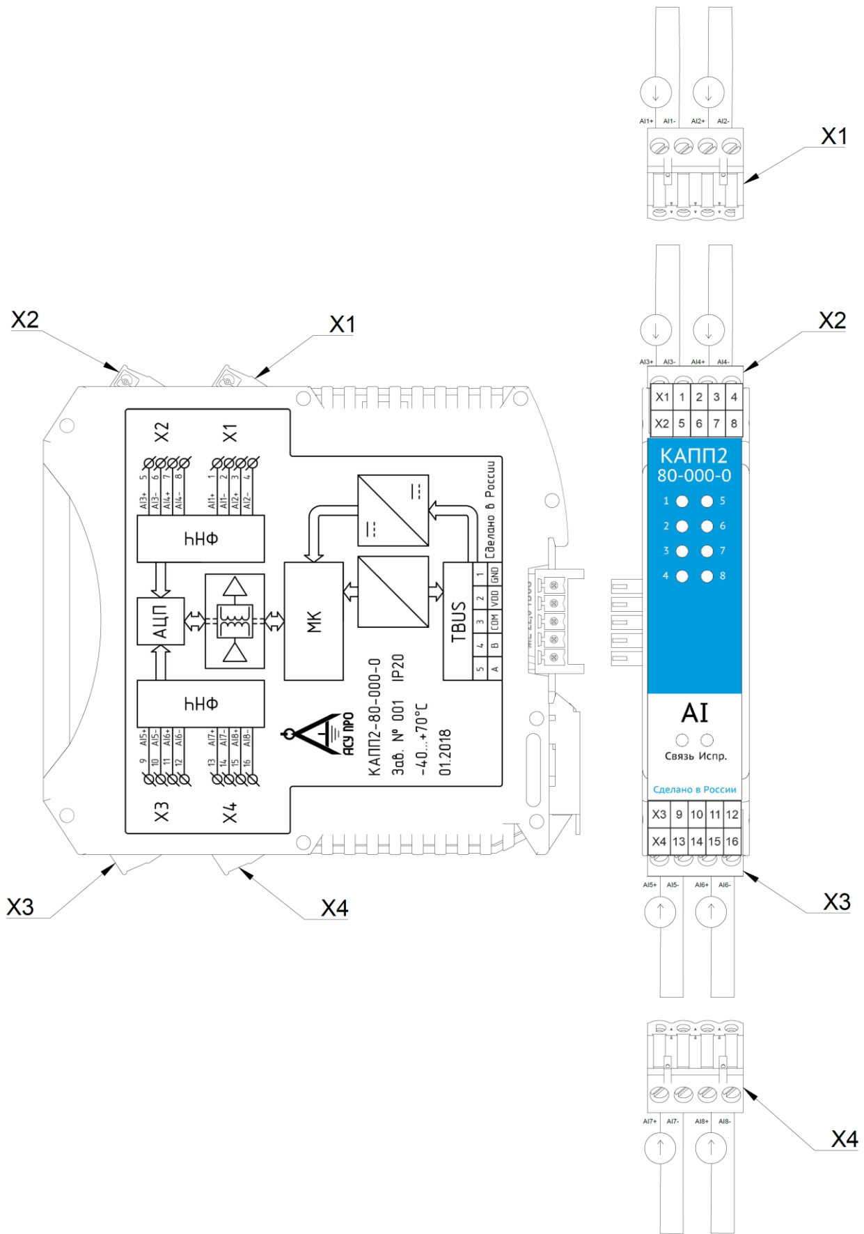
Рисунок 3 – Схема соединений модуля КАПП2-80-000-0 в режиме измерения напряжения
