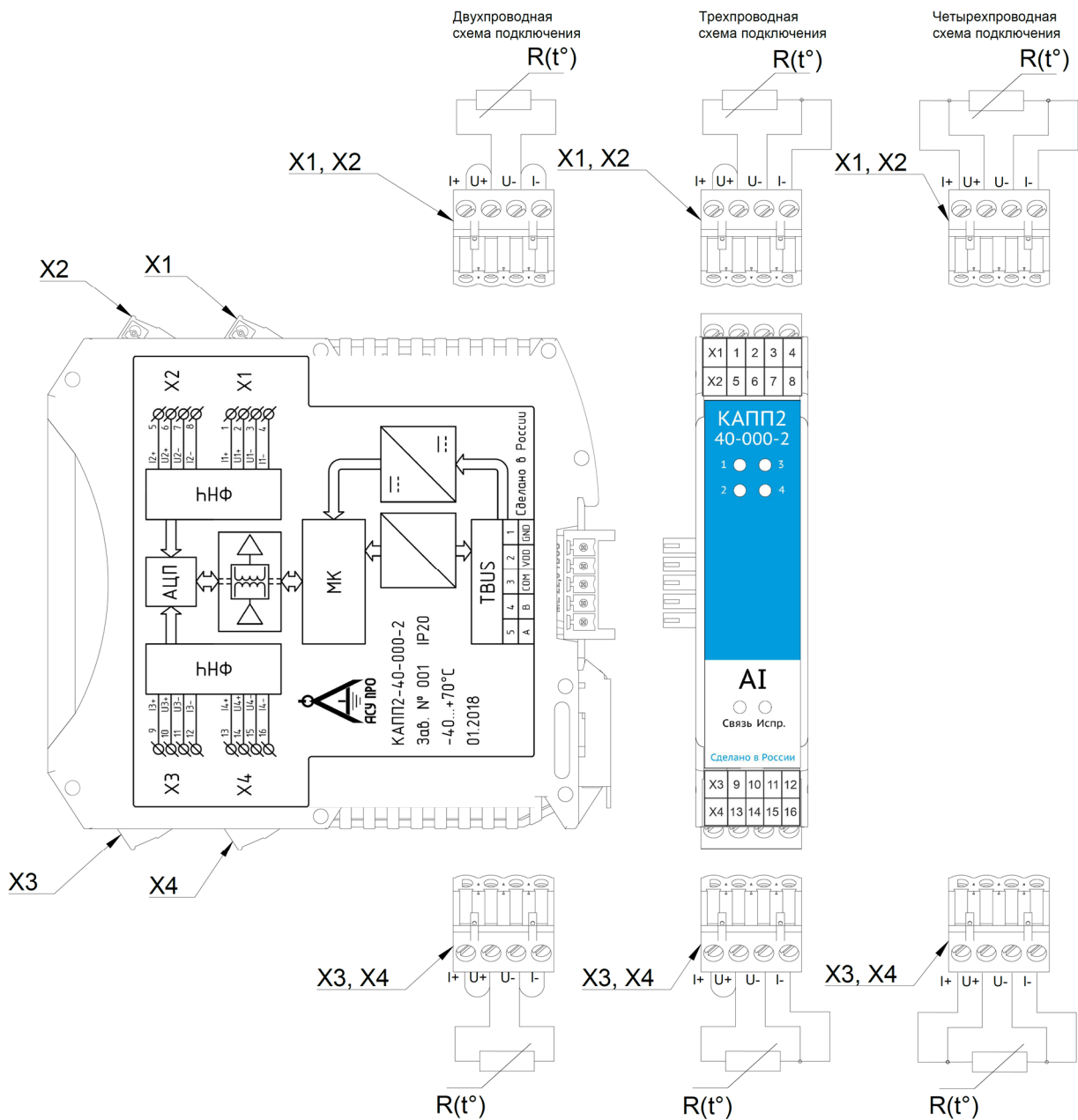
Рисунок 3 – Схема соединений модуля КАПП2-40-000-2 для работы с термопреобразователями сопротивления
