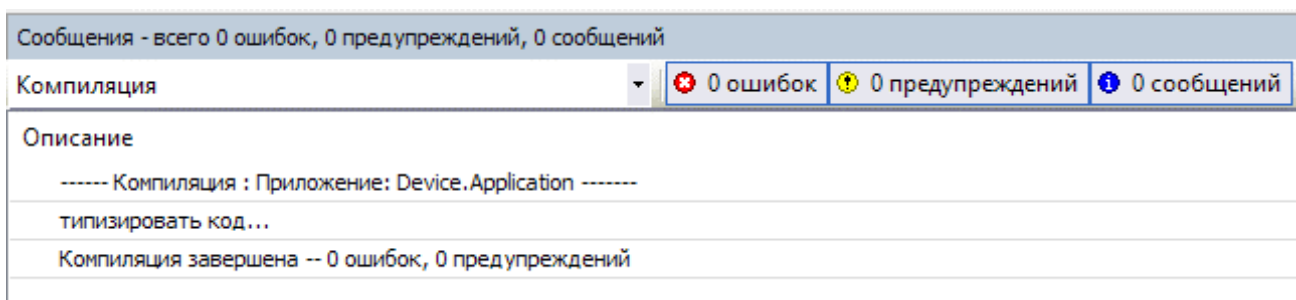
Рисунок 47 – Результаты компиляции
