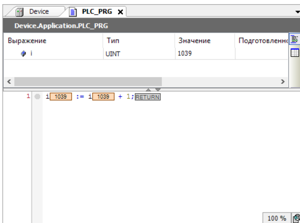
Рисунок 54 – Выполнение программы
