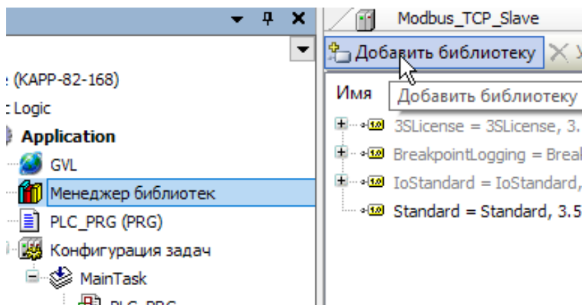
Рисунок 69 – Менеджер библиотек
