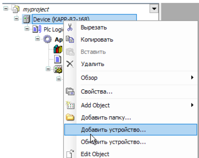
Рисунок 55 – Добавление устройства
