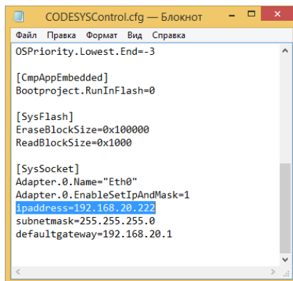
Рисунок 88 – Содержание конфигурационного файла CODESYSControl.cfg Так же стоит учитывать, что у контроллера КАПП-82-168 один порт Ethernet. Работы с регистрами Modbus осуществляется так же, как и в случае драйвера Modbus RTU Slave пункт 2.4.3.
