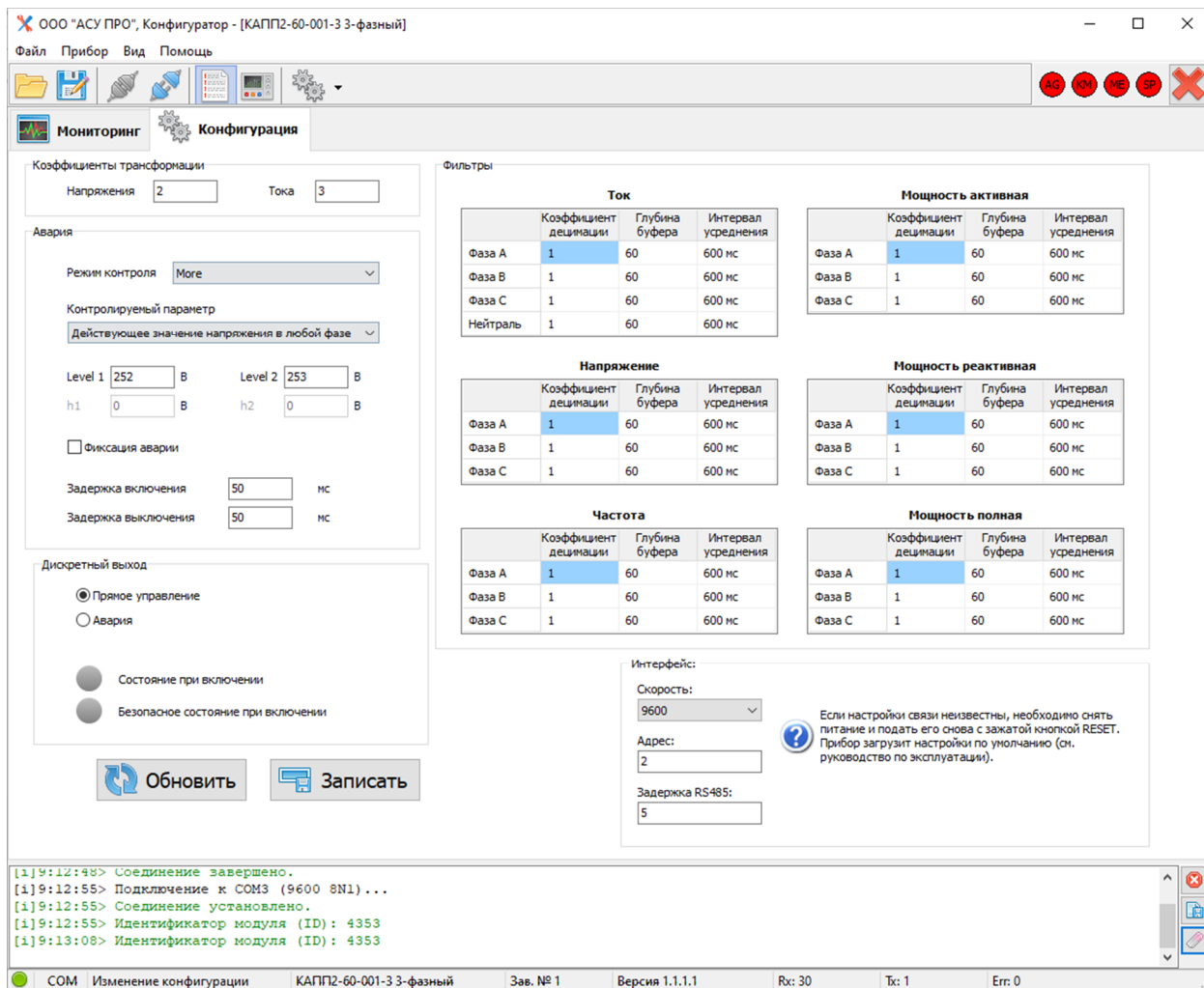
Рисунок 10 - Изменение конфигурации
