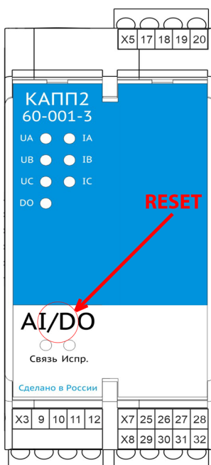
Рисунок 12 – Расположение кнопки «RESET»
