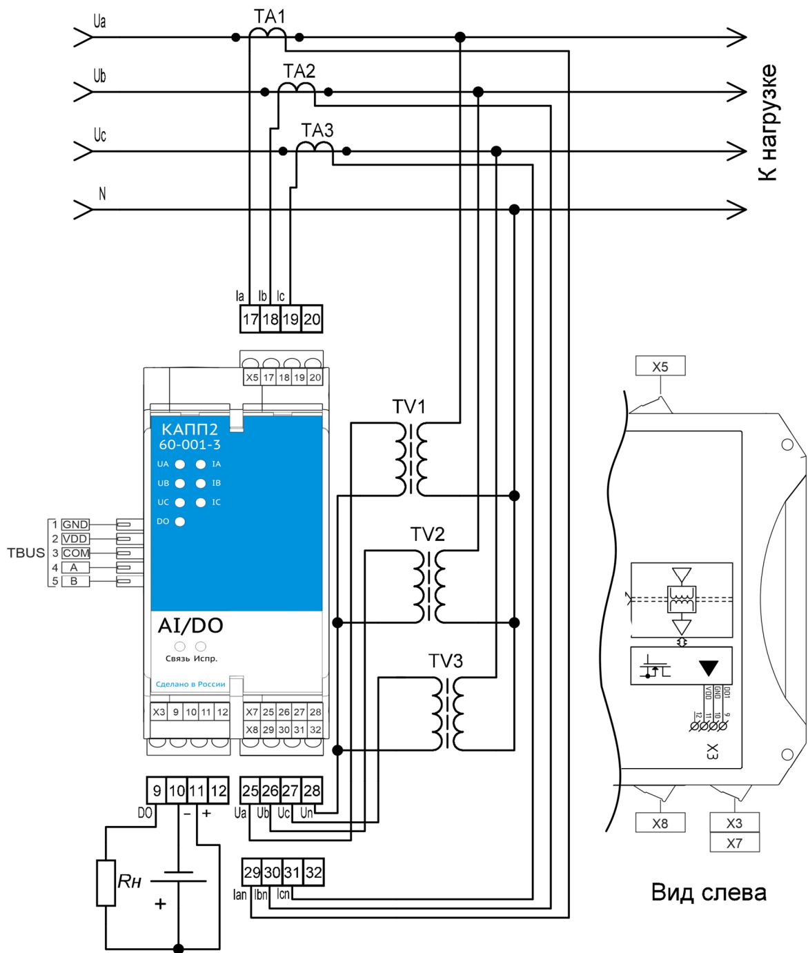
Рисунок 3 – Схема соединений модуля КАПП2-60-001-3 при подключении через согласующие трансформаторы
