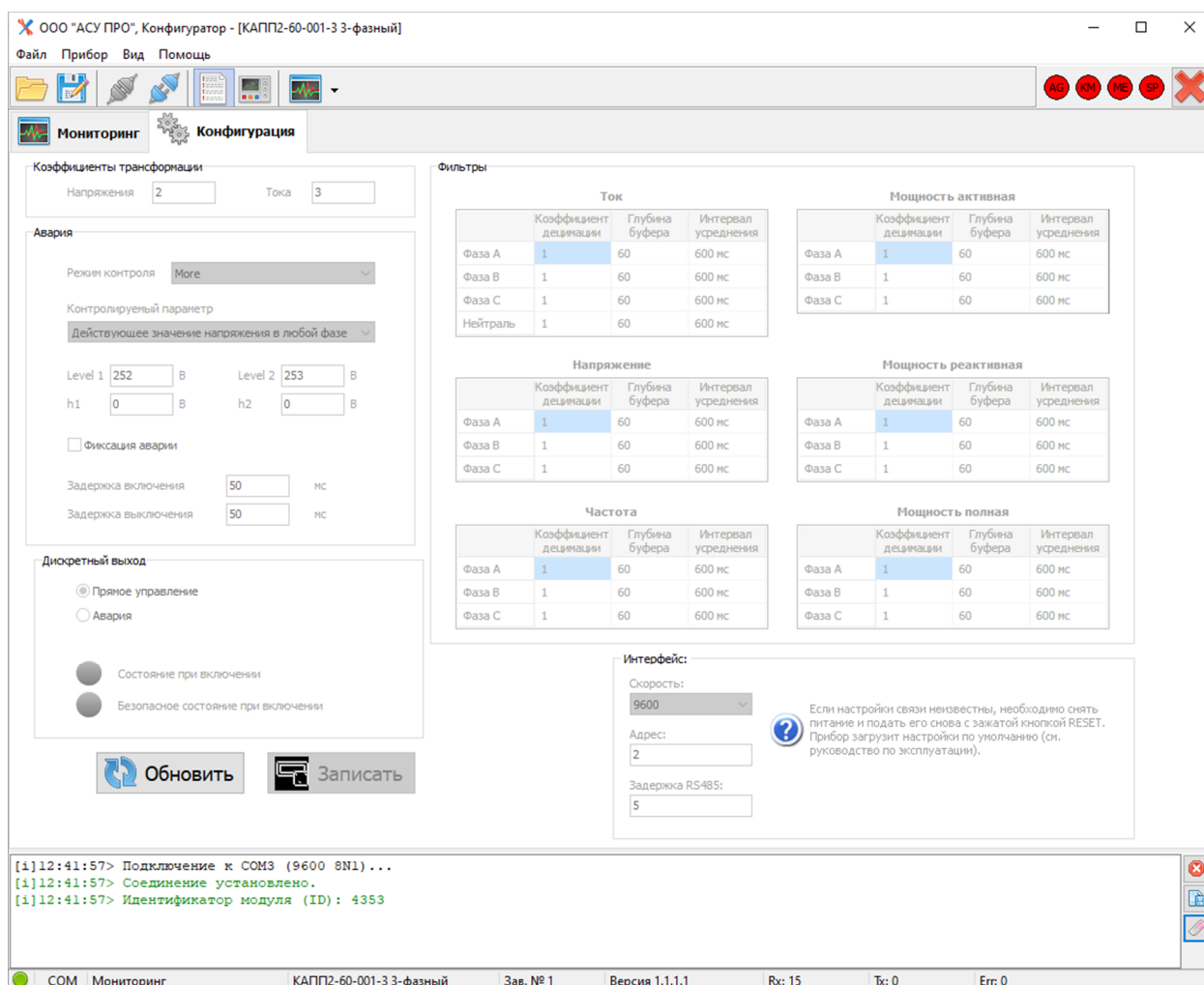
Рисунок 9 – Окно конфигурации
