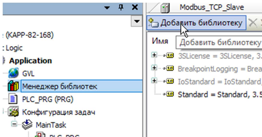
Рисунок 64 – Менеджер библиотек
